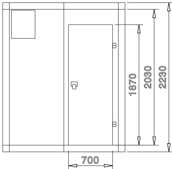
Zij aanzicht
